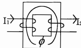
図1. 従来型(内鉄型)変圧器の構成
