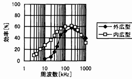
(a)フラット型変圧器 (a) Film transformer
